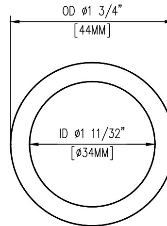
TOP VIEW SCALE: 1:1
